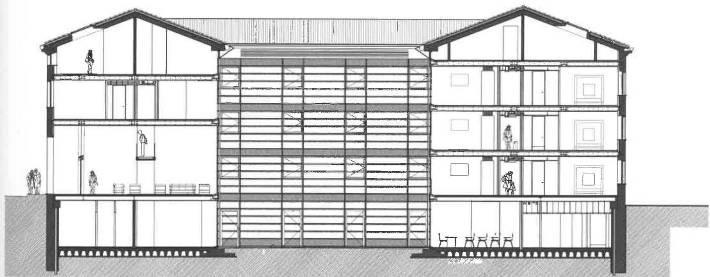
Sección CC
