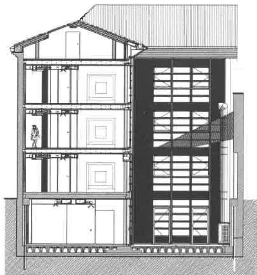
Sección BB
