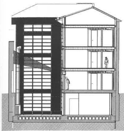
Sección AA
