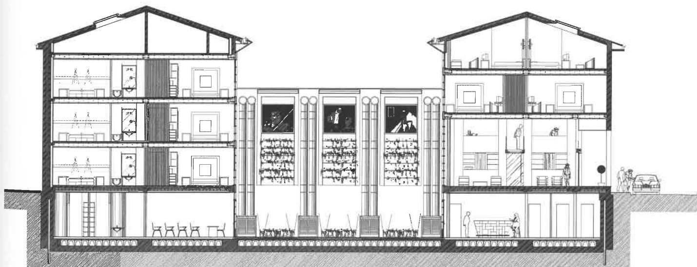
Sección DD
